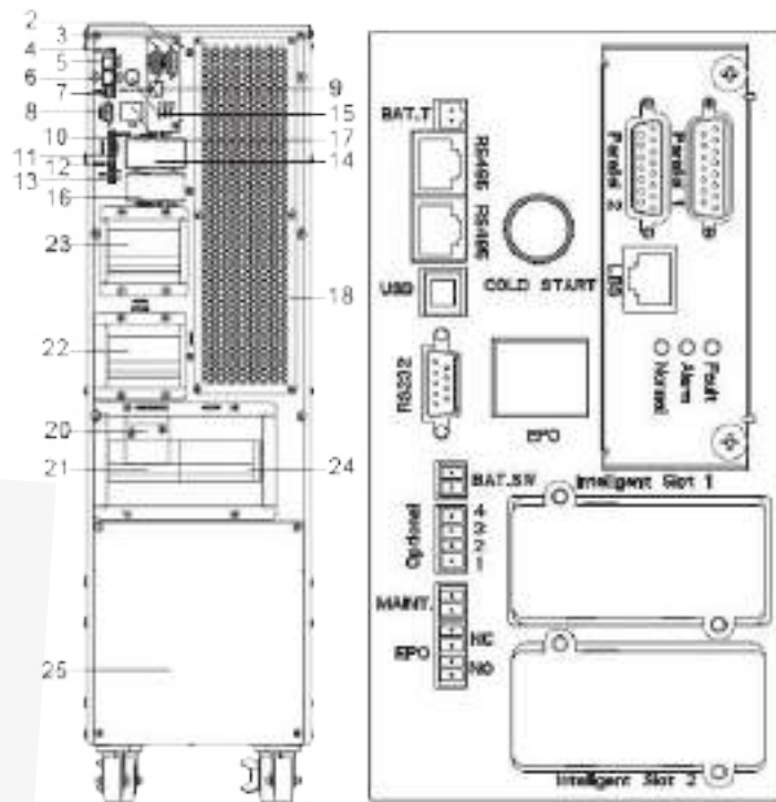
Vista trasera
