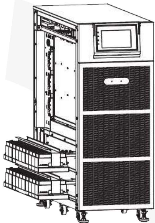
Lado izquierdo del gabinete (extraiga la batería)
