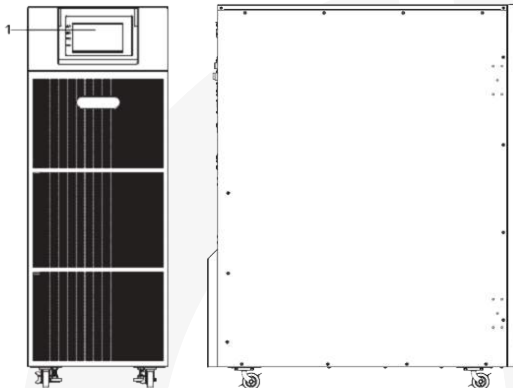
Vista frontal / Vista lateral
