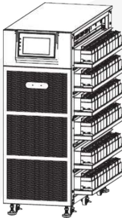
Lado derecho del gabinete (extraiga la batería)
