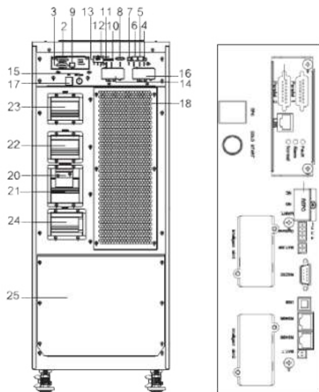
Vista trasera
