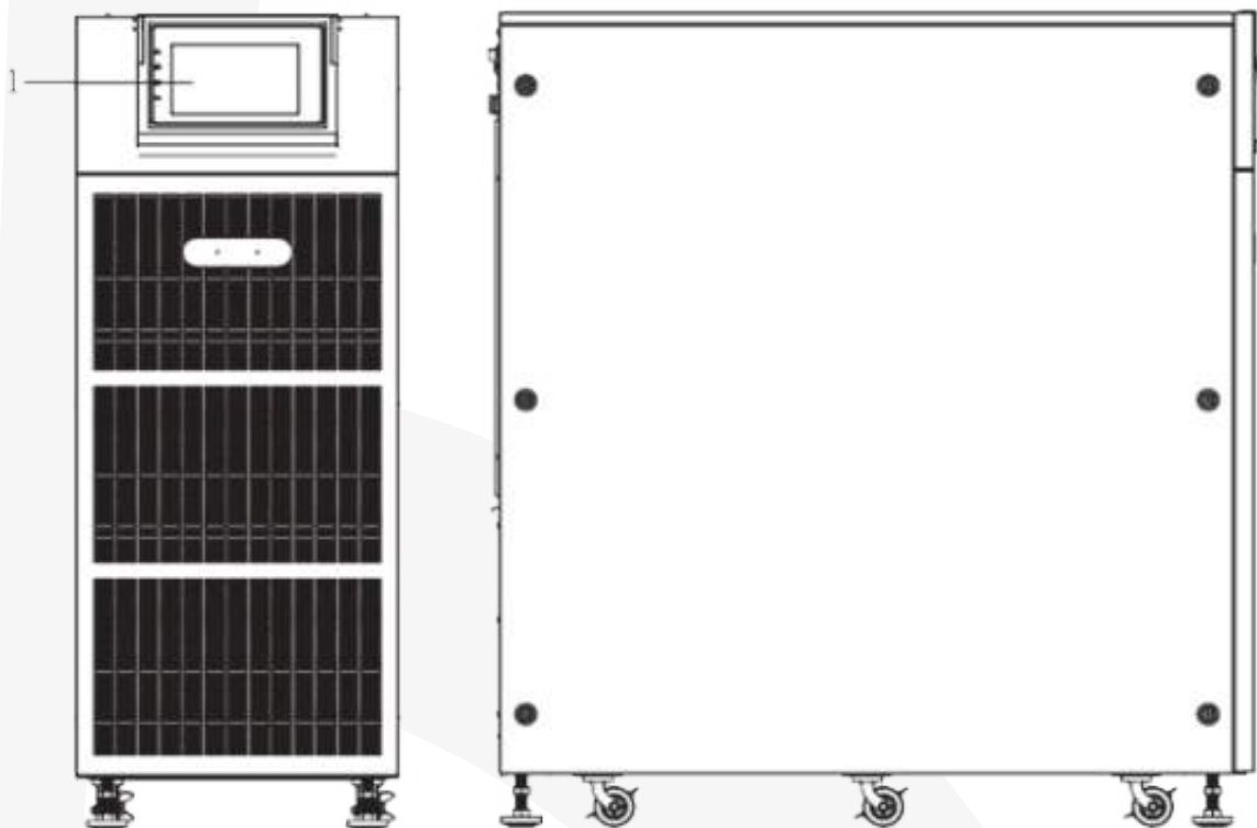
Vista frontal / Vista lateral
