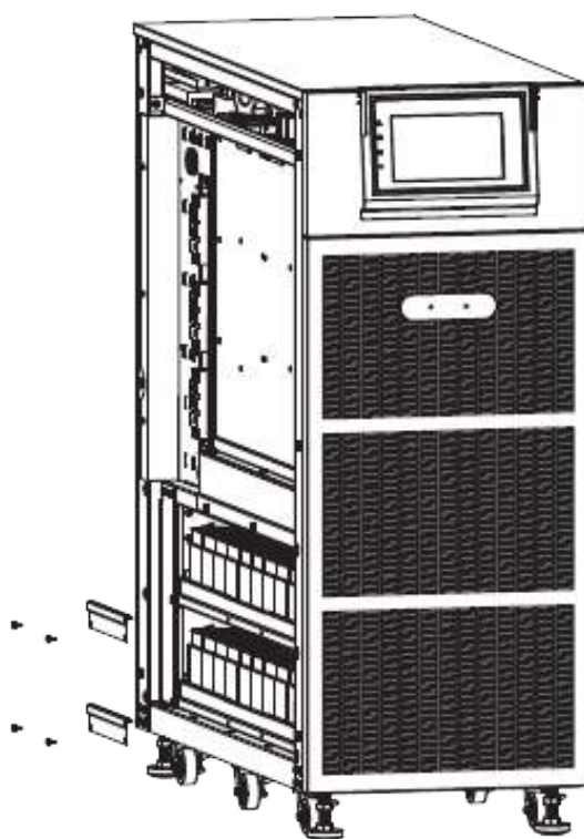
Lado izquierdo del gabinete (quitar tornillos y cubiertas)
