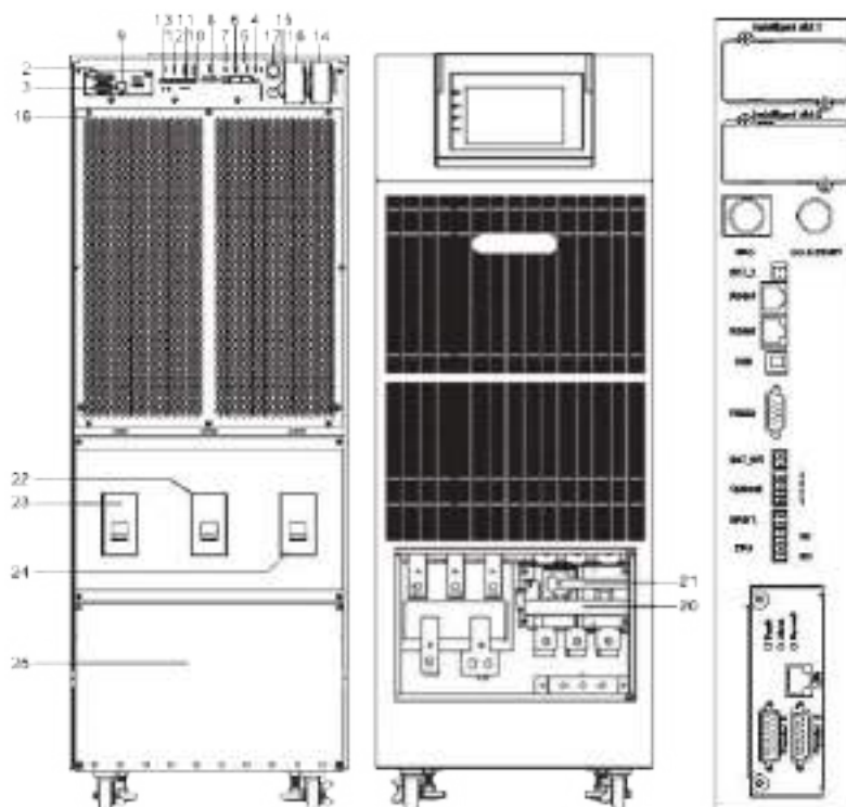
Vista trasera
